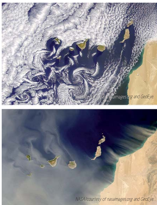
Figura 1. Las islas Canarias están expuestas a los vientos alisio del Noreste (arriba) y sahariano (abajo). Obsérvese, por una parte, cómo las islas interceptan la humedad y el polvo transportados, respectivamente, por dichos vientos; por otra, las perturbaciones (vórtices) que provocan en el flujo de aire cuando éste es obstaculizado por las islas.
