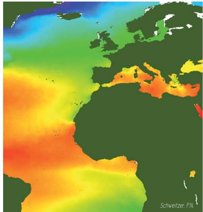
Figura 2. Temperatura superficial del mar en el mes de agosto calculada a partir de datos recogidos por satélite (NOAA-AVHRR, promedio del periodo 1981-1990). Nótese la "anomalía" del gradiente latitudinal que se produce en el entorno de las islas Canarias como consecuencia de la corriente fría de Canarias y del afloramiento de aguas profundas en la costa sahariana. (Schweitzer, P.N. 1993. Modern Average Global Sea-Surface Temperature: U.S. Geological Survey Digital Data Series DDS-10, U.S. Geological Survey, Reston, Virginia)
